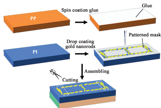
图2 双层软体致动器制备过程
