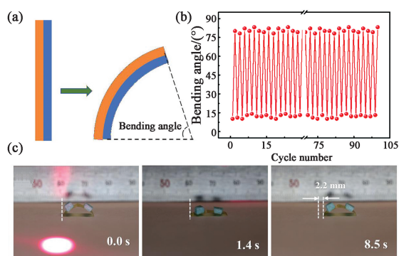
图5 基于金纳米棒的软体致动器。(a)弯曲原理;(b)808 nm激光激发循环次数;(c)负重软体爬行机器人。
