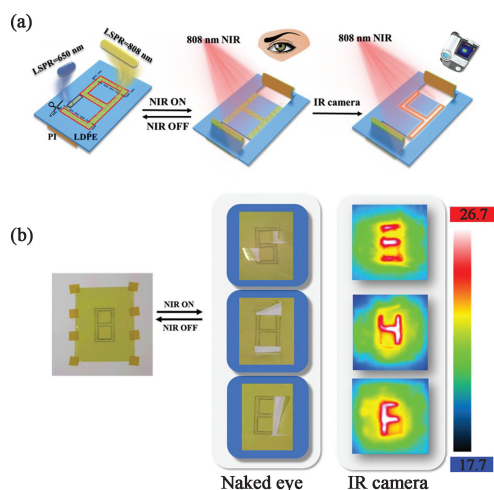
图 6 基于软体致动器的信息示假隐真技术。(a) 信息示假隐真技术的示意图;(b) 不同类型的信息示假隐真图片。
