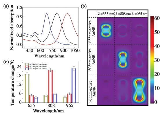
图 4 不同金纳米棒的表征。(a)紫外可见吸收图谱;(b)FDTD 模拟金纳米棒周围电场强度;(c)不同长径比金纳米棒在不同激光下最大的光热。
